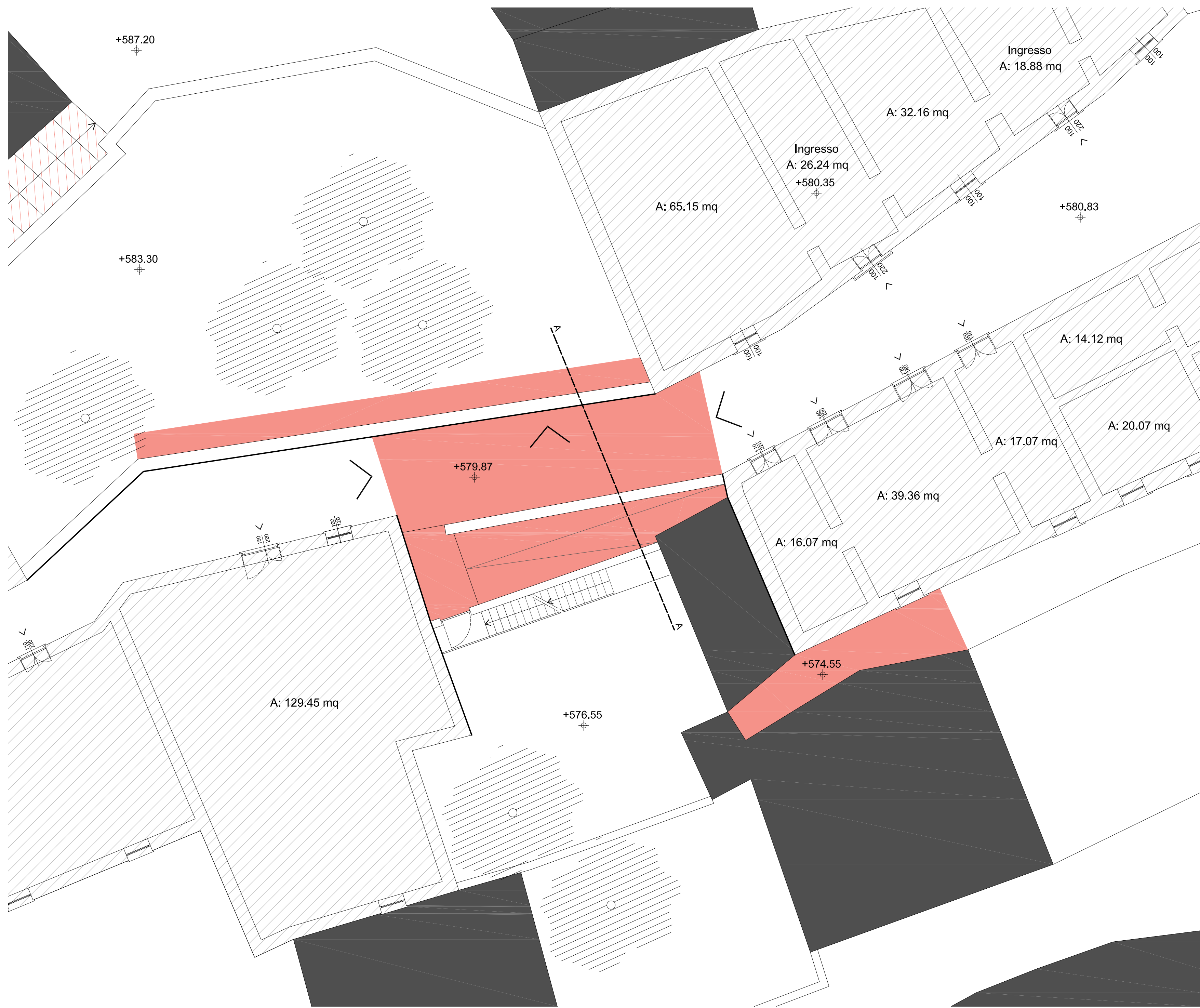
C_luogo notevole Scala 1:100 Incontro tra Corso Mazzini e una rampa coperta
