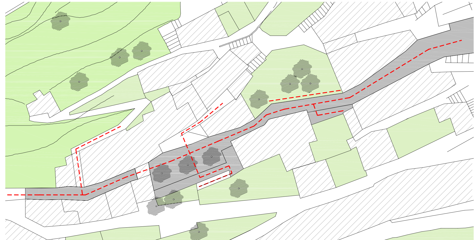
Stralcio planimetria Spazi Verdi Scala 1:500
