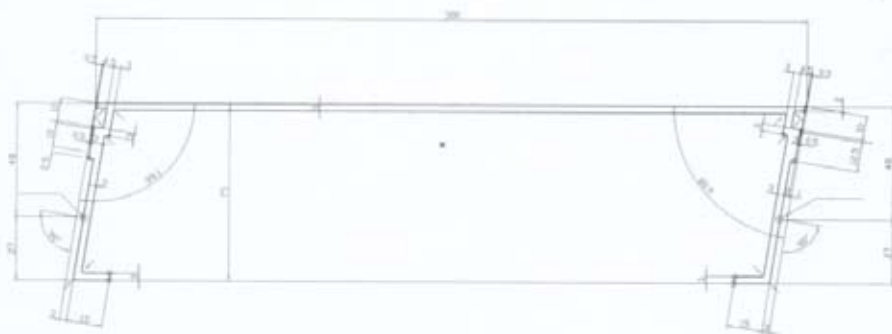
Panel de cerramiento y suelo / Wall-floor panel
