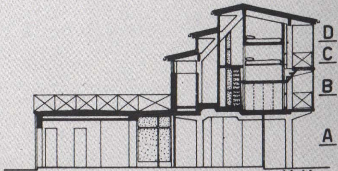
SEZIONE TRASVERSALE X-X
