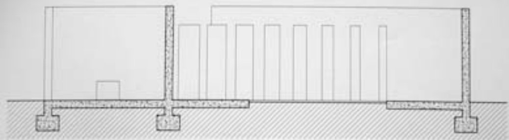
Sezione A-A
